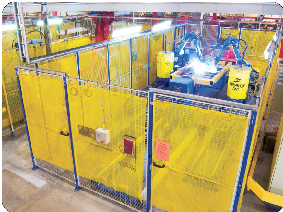
X-Guard tillsammans med svetsdraperier skyddar mot kläm- och brännskador samt skadlig UV-strålning.
