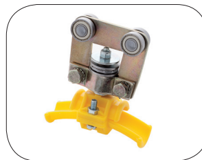
KABELVAGN FÖR RUNDKABEL, ROTTERANDE Ø 10-16 mm – Artnr 521019 Ø 17-25 mm – Artnr 521020 Ø 26-36 mm – Artnr 521021
