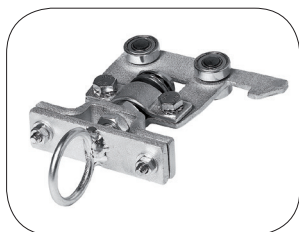
VAGN MED VRIDBAR ÖGLA OCH HAKE Artnr 521006
