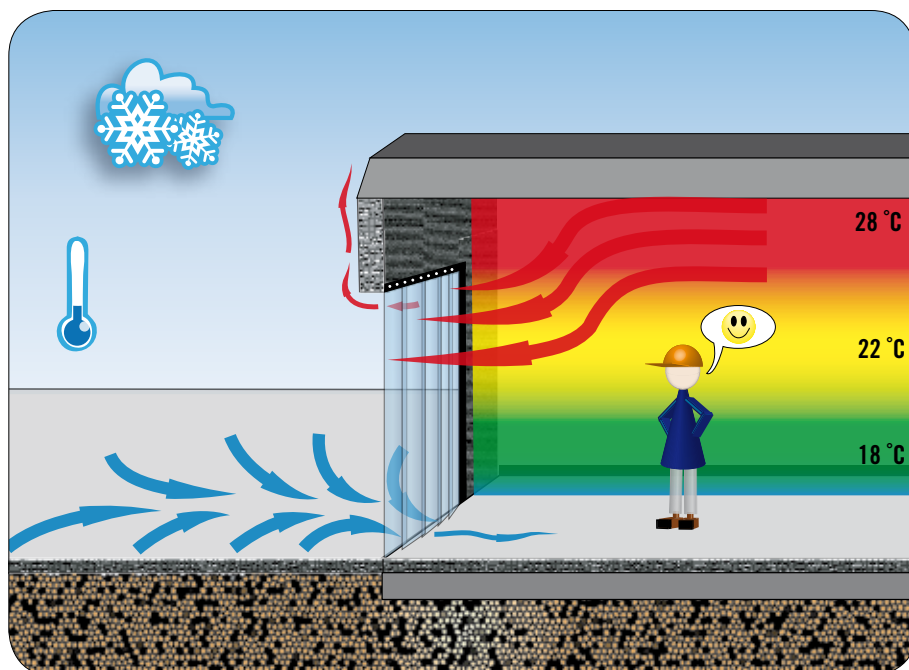
Varm- och kallluftsflöde med Multiporten.
